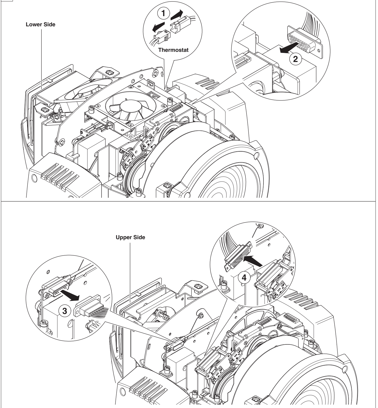
Estrazione moduli effetti: Operazioni preliminari - Figura 16
